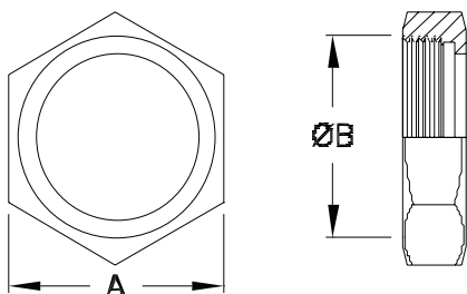
Nut
