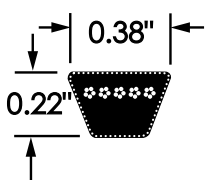
83 3L SECTION
